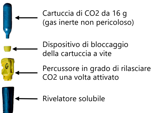
Fig 6: Diverse parti dell'attivatore
