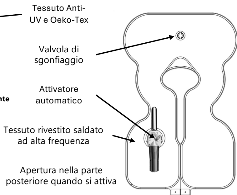
Fig 4: Disegno della parte gonfiabile
